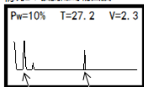
障碍物回波 液面回波
