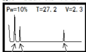
管口回波 管口二次回波 液面回波
